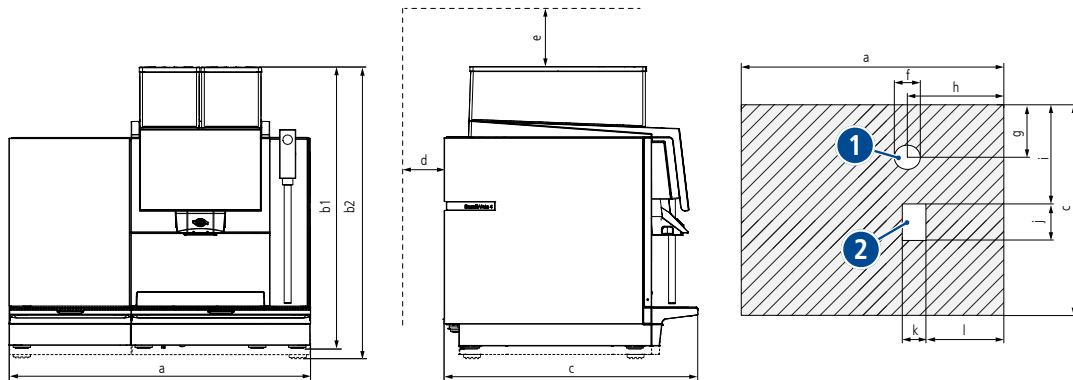
1 Ausschnitt für Wasser-/Milcheingang und Wasserablauf. Auch für Netzkabel möglich. 2 Ausschnitt für Satzabwurf
